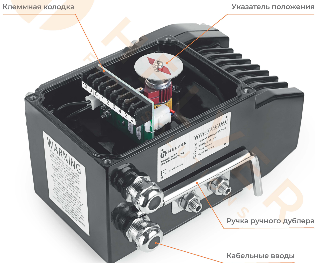
Рисунок 1 – Внешний вид и основные элементы привода
