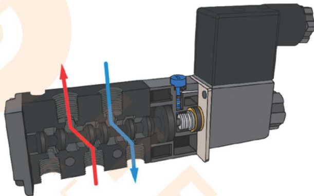
Рисунок 1 – Положение клапана до подачи напряжения
