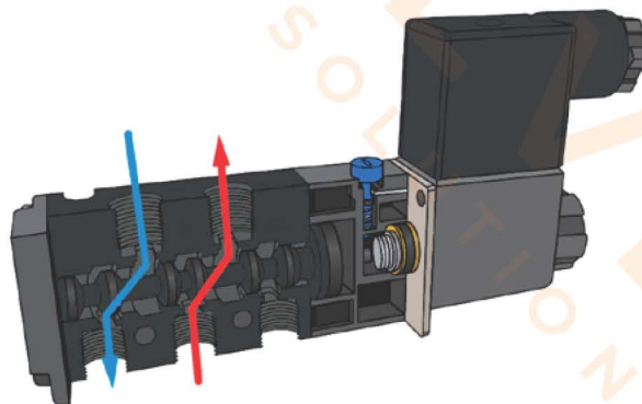
Рисунок 2 – Положение клапана после подачи напряжения
